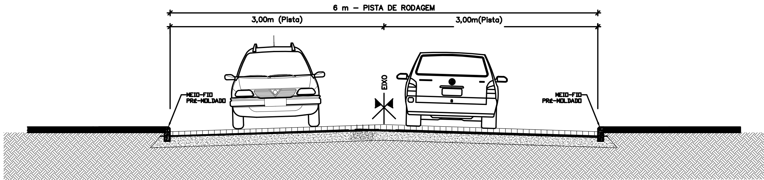
SEÇÃO TIPO DE BLOCO INTERTRAVADO - ESTRADA LINHA SARAIVA
